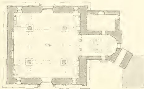
Kirche zu Mongiovino.
